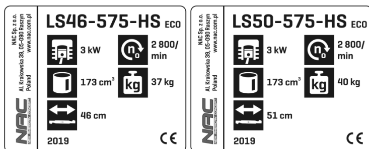
Tabliczka znamionowa
